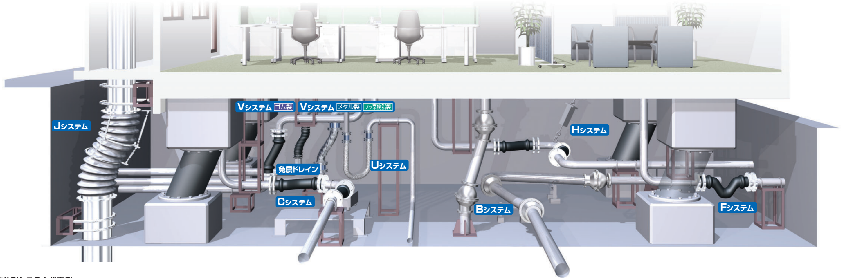
流体別システム代表例 ※下表は代表例です。選定時にはご相談ください。 ※免震継手の材質についてはP.11を参照してください。
